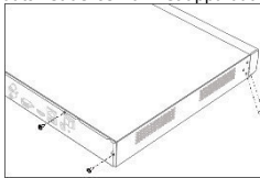
Figure 2-1 Verwijder het deksel
