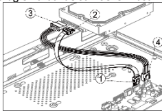
Figure 2-2 Verbind de kabel
