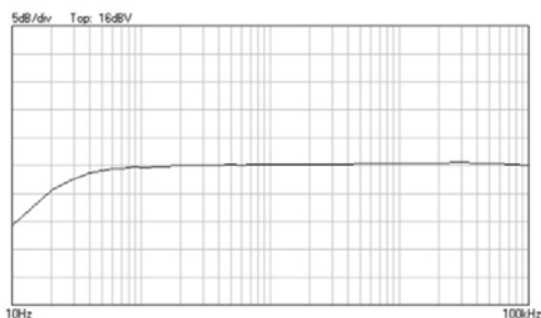
Risposta in frequenza su 8 ohm
