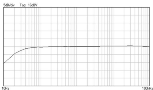
Réponse en fréquence @ 8 ohms
