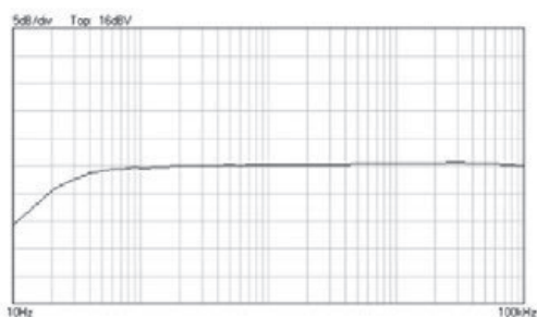
Taajuusvaste @ 8 ohmia
