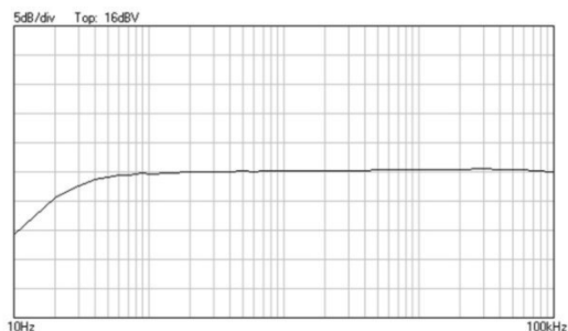
Respuesta en frecuencia @ 8 ohm
